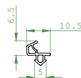
Rubber Gasket (Sash) : Code: 34024-12010
